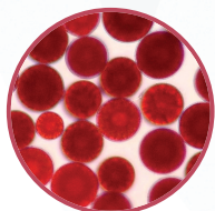
虾青素 ASTAXANTHIN
